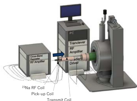
アドオン型 ^1\text{H}/^{23}\text{Na} ハイブリッドMRIシステムとライブマウスイメージングの例
