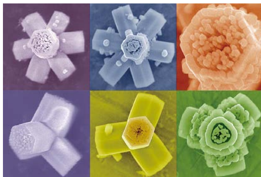
ZnS/SiO混合物を窒素雰囲気中で1300°C加熱して得られた6回対称7脚構造と3回対称4脚構造のZnS ナノフラワースのSEM像 SEM images of 6-fold symmetry heptapod-and 3-fold symmetry tetrapod-like ZnS nanostructures fabricated by thermal evaporation of a ZnS and SiO mixture source in N 2 at 1300°C
